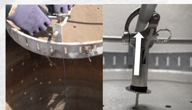
6. Schmutzfänger wieder einsetzen und Seil von unten in das Seilschloss einfädeln. Zum Entriegeln der Seildurchführung Druck auf die untere Scheibe ausüben.
