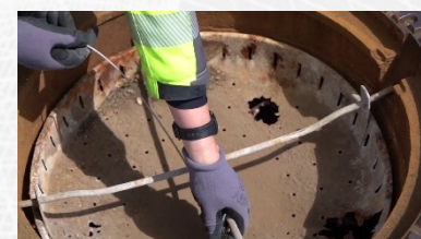
7. Jetzt das Seil durch das Seilschloss straffziehen bis das Gewicht der Rattenkugel zu spüren ist (Rattenkugel muss auf der Berme stehen bleiben). Das Seilschloss fixiert automatisch das Seil.
